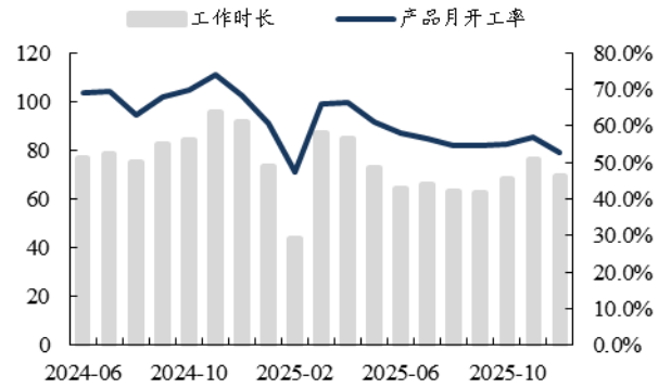
图6: 2025年12月国内挖机开工69.3小时,同比-24%
