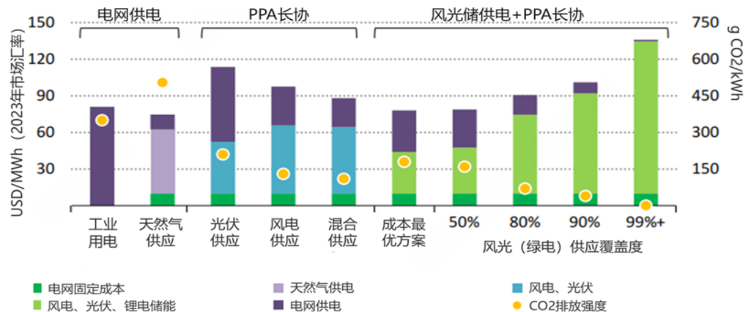
2024年美国数据中心不同供电组合LCOE及碳排放强度
