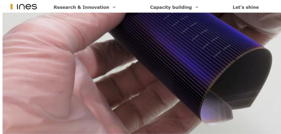
图：法国国家太阳能研究所已研发出60 μm柔性太空用HJT电池可实现柔性设计，满足特殊卫星结构
